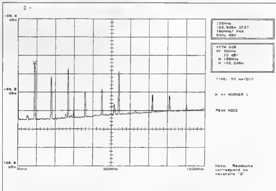
Figuur 3: De stoorprodukten op de antenne-aansluiting.
